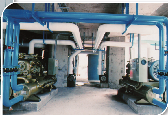
350噸冰水設備
